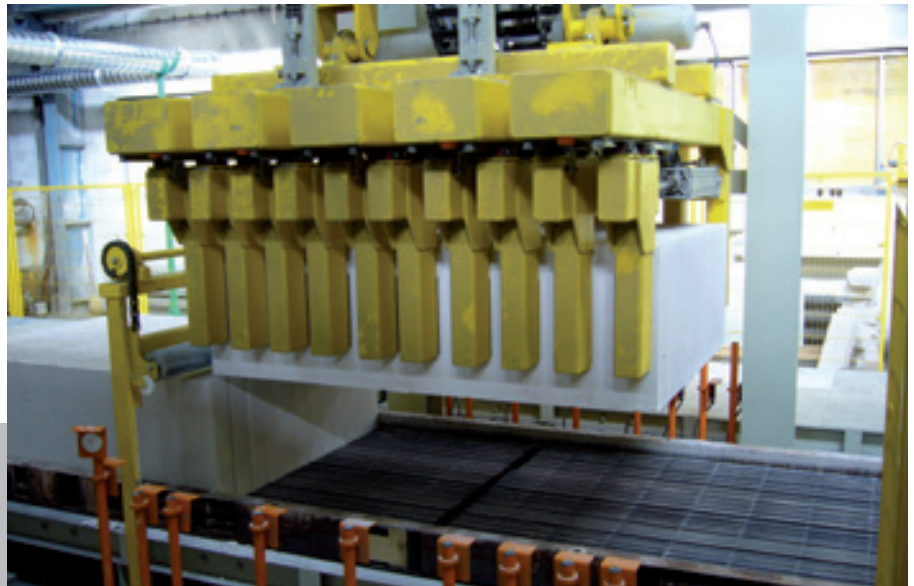
Blockumsetzer Перестановщик блоков
